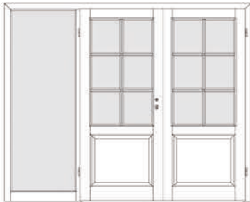
WID1S 2-flgl. Tür mit 1 festen Seitenteil links
